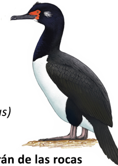
Cormorán de las rocas Magellanic (Rock) cormorant ( Phalacrocorax magellanicus )
